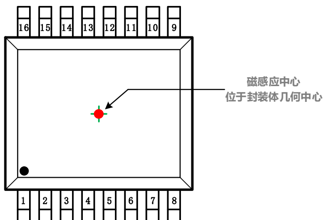
图-1: MT6835 TSSOP-16封装外观图
