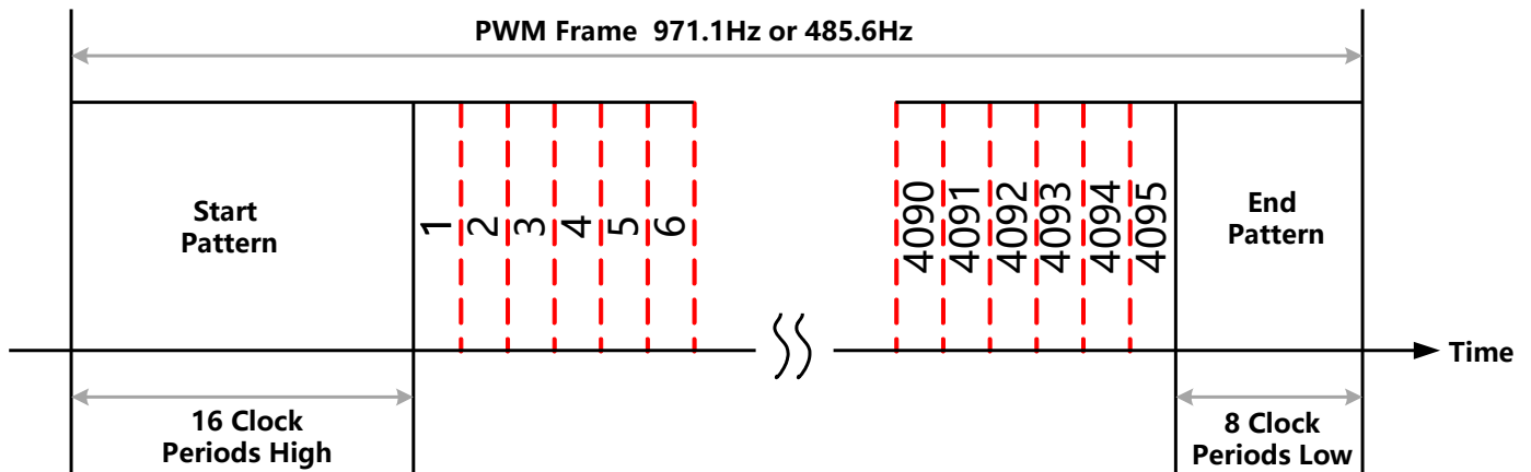
图-13: PWM输出
