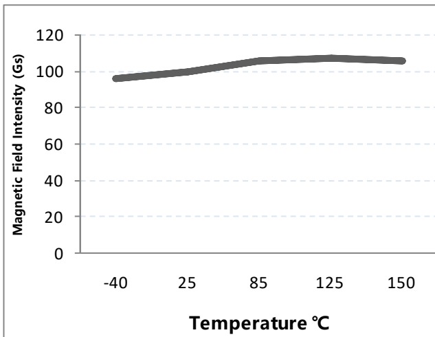
图.8 磁特性 vs. 温度 (BHYS)
