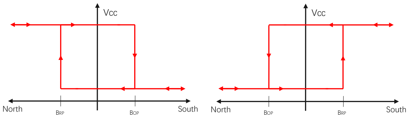
图.2 Flat TO-92 & SOT-89-3L & SOT-23 (ThinOutline) 的开关功能
