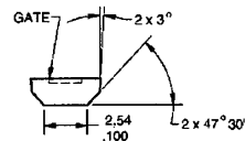
标准引脚
