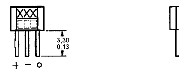
短脚(-R)
