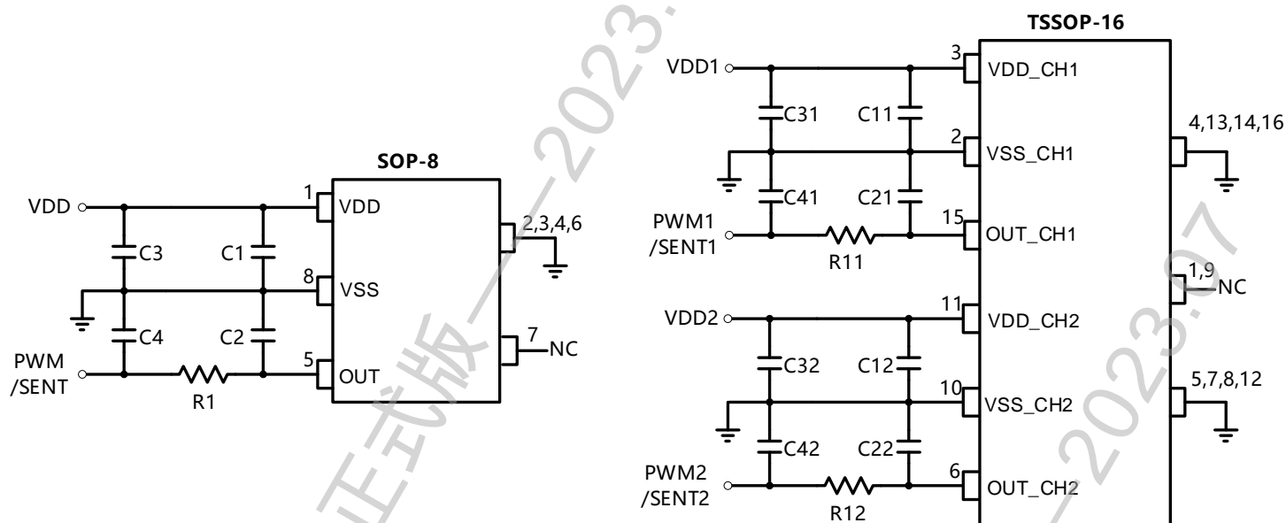
图-29: PWM、SENT推挽输出模式参考电路
