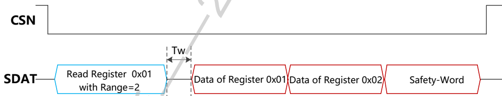
图-16: SPI 读当前角度数据
