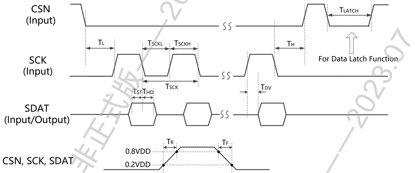
图-11 3线SPI时序图
