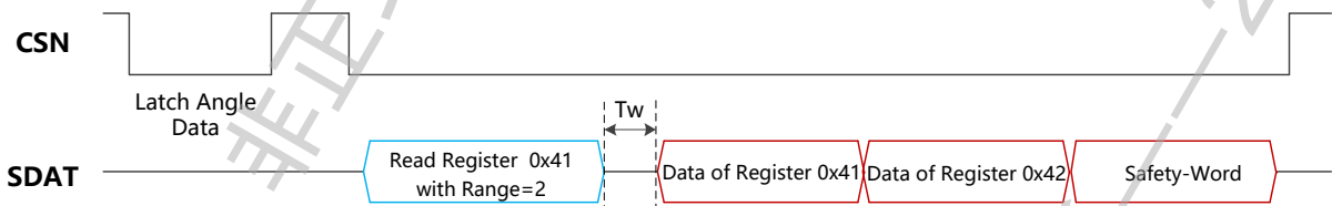
图-17: SPI 读锁存角度数据
