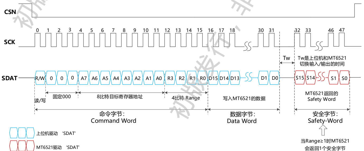
图-13: 3线SPI写操作
