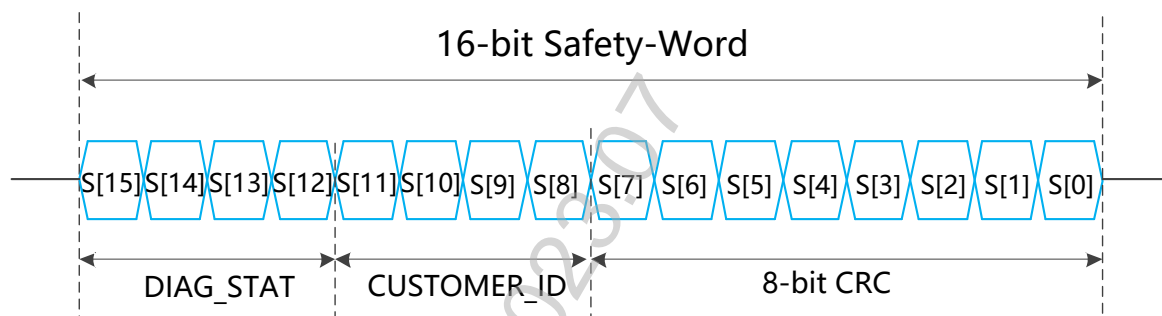
图-15: 安全字结构
