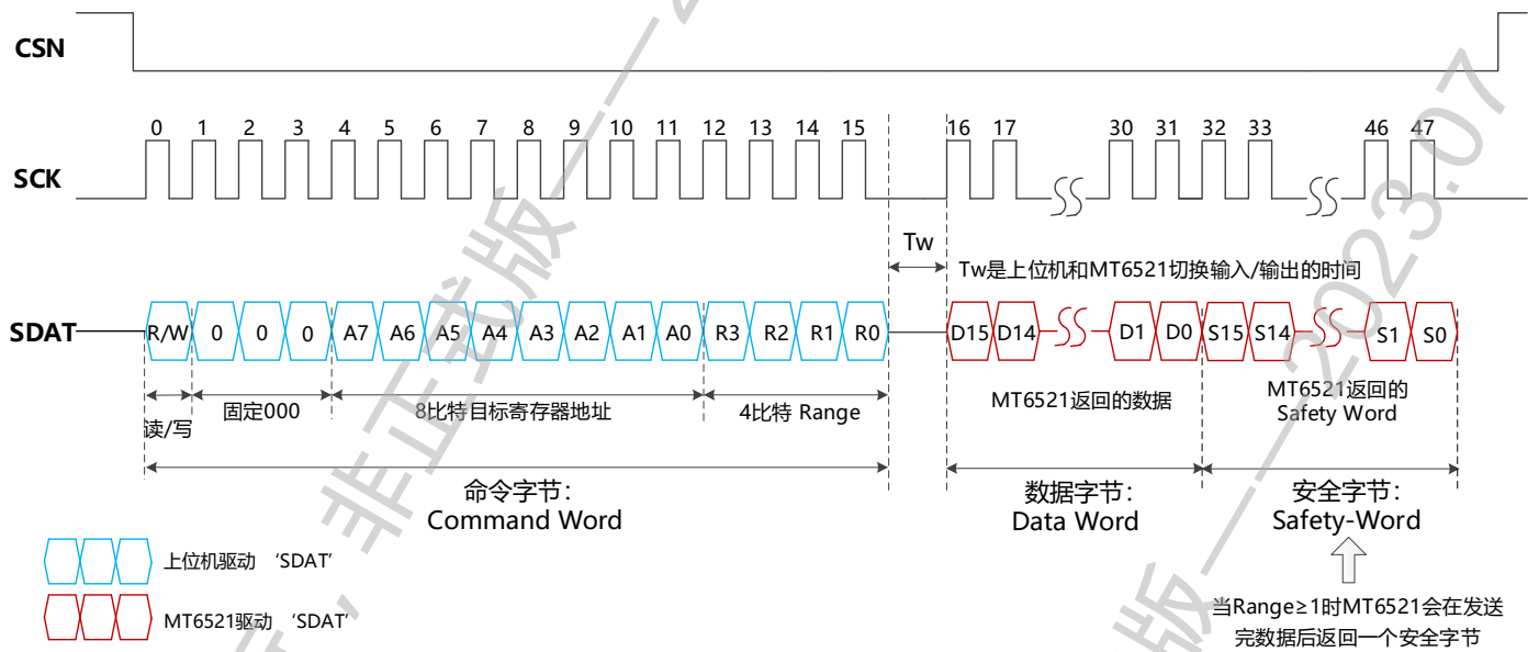
图-12: 3线SPI读操作
