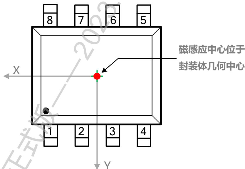
图-1: SOP-8封装
